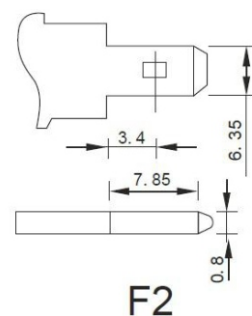
Złącze akumulatora
