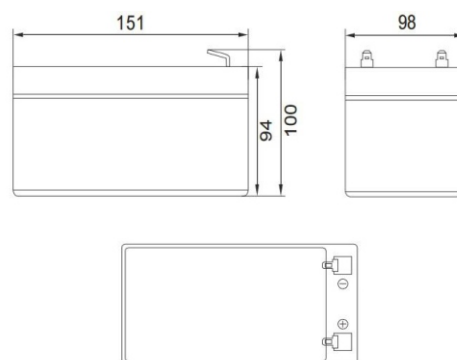
Wymiary
